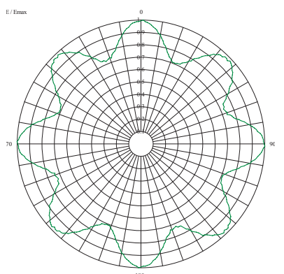
HRP HPOL PCP500-D 1.30dBd
