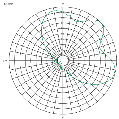
HRP VPOL PCP500-B 4.06dBd
