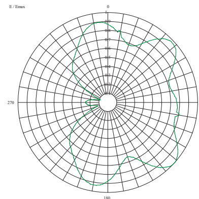
HRP VPOL PCP500-C 2.9dBd
