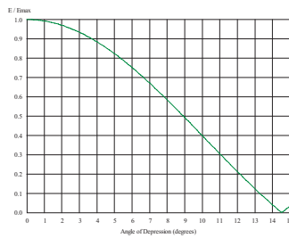
VRP VPOL PCP500-2 6.54dBd
