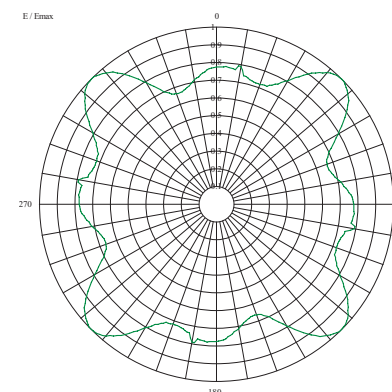
HRP VPOL PCP500-D 1.9dBd
