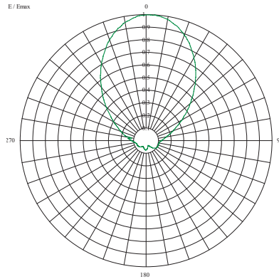
HRP VPOL PCP500-A 7.14dBd
