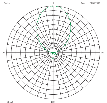
HRP HPOL PCP500-A 7.4dBd
