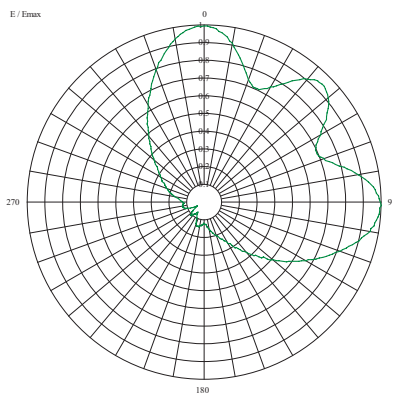
HRP HPOL PCP500-B 4.6dBd
