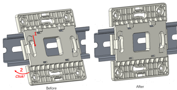
Din 35 mounting
