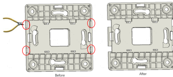
Din 35 mounting
