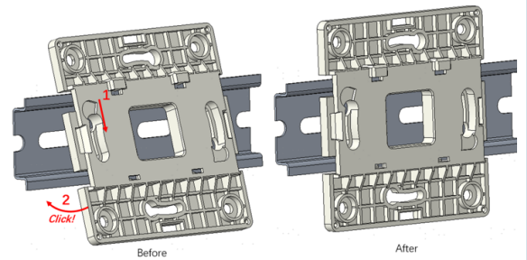
Din 35 mounting
