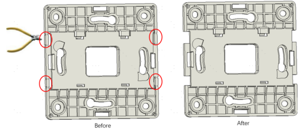
Din 35 mounting
